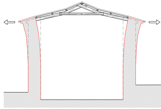
▲ Fig. 6: Esquema das deformacións producidas nos muros por un deterioro da estrutura da cuberta. Elaboración propia.
