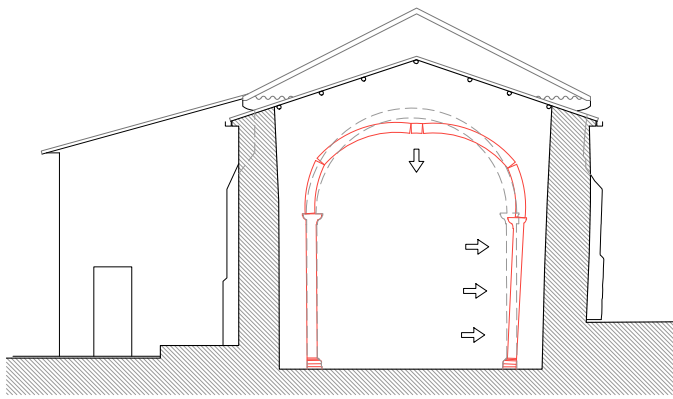
▲ Fig. 5: Hipóteses do desplome do arco toral. Elaboración propia.
