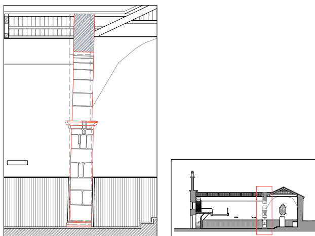
▲ Fig. 7: Deformación da pilastra norte de apoio do arco toral. Nótase a inclinación cara a zona leste, correspondente co presbiterio. Elaboración propia.
